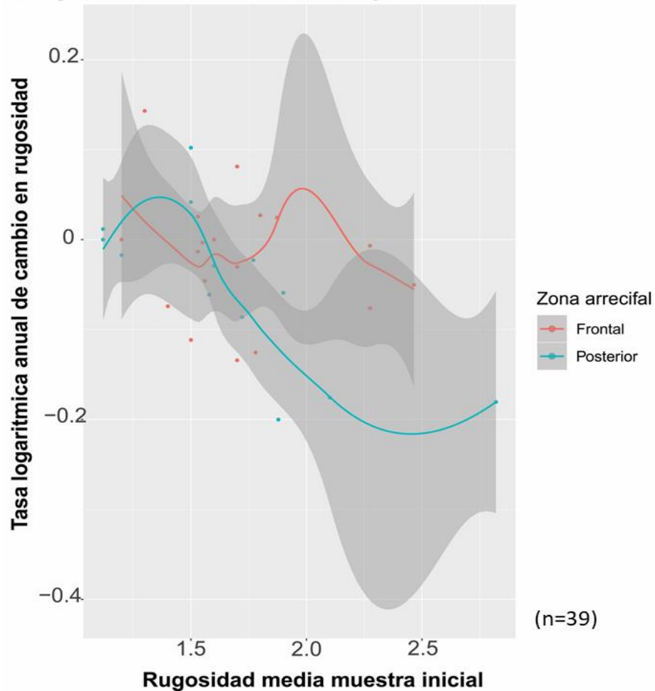
Tasa logarítmica anual de cambio en rugosidad vs rugosidad media muestra inicial y zona arrecifal.
